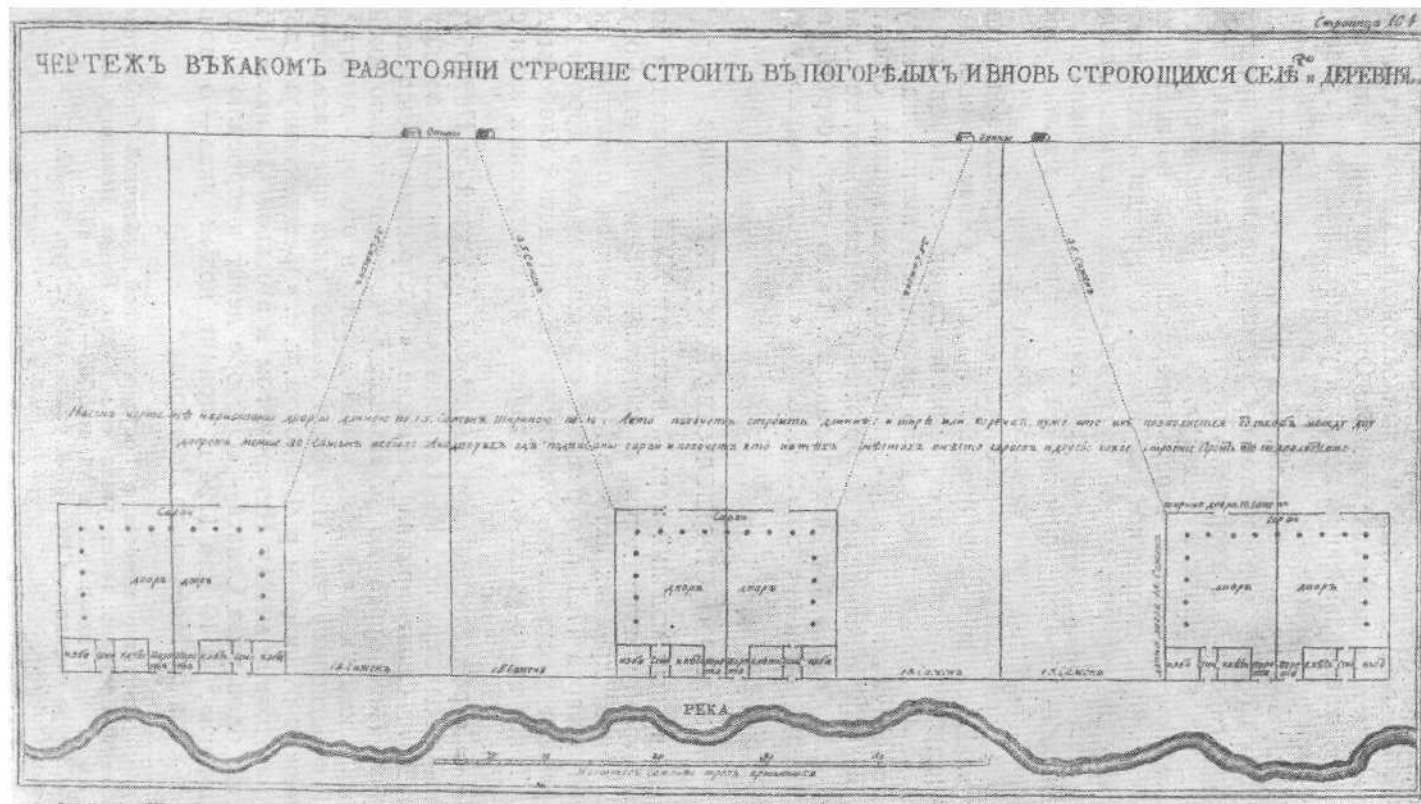
Рис. 106. «Чертеж, в каком разстоянии строение строить в погорелых и вновь строящихся селех и деревнях», приложенный к указу о противопожарной планировке крестьянских дворов. (1722 г.).
