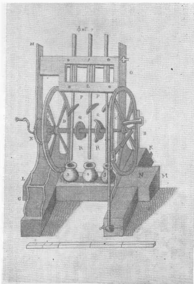
Рис. 60. Пороховая мельница: толчея и бегуны. Чертежи из книги «Учение и практика артиллерии». (1711 г.).
